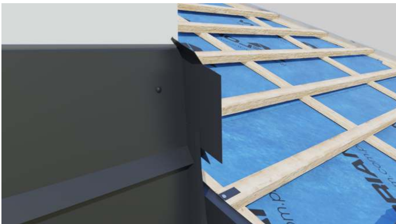
Arkusz powinien posiadać zakład z przodu i z tyłu komina - z przodu, aby możliwe było zaklepanie na przednią obróbkę i z tyłu, aby można było na niego zaklepać obróbkę tylną.
