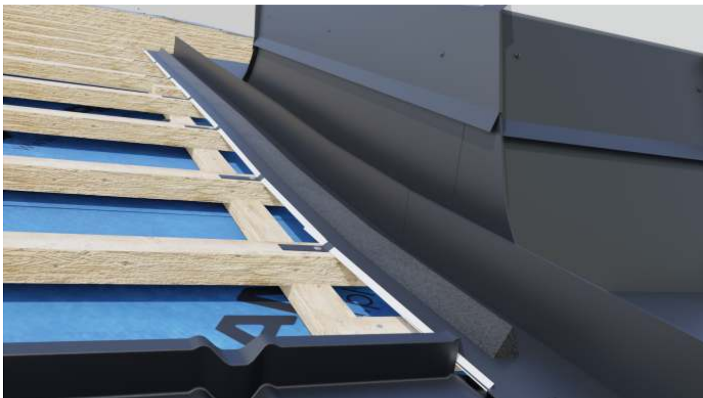
Na obróbkę naklejamy uszczelkę klinową.
