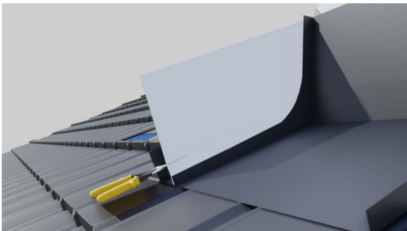
Obróbkę w przedniej części obcinamy pod kształt obróbki przedniej pozostawiając około 1 cm marginesu.
