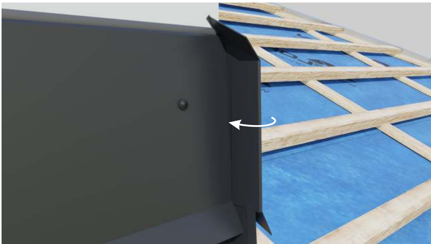
Zaklepanie obróbki bocznej z przodu.
