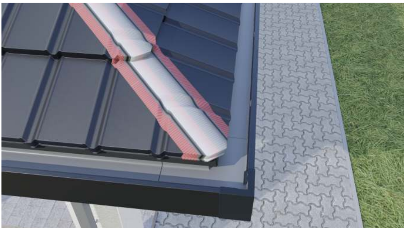
Taśma przyklejona do dachówek.
