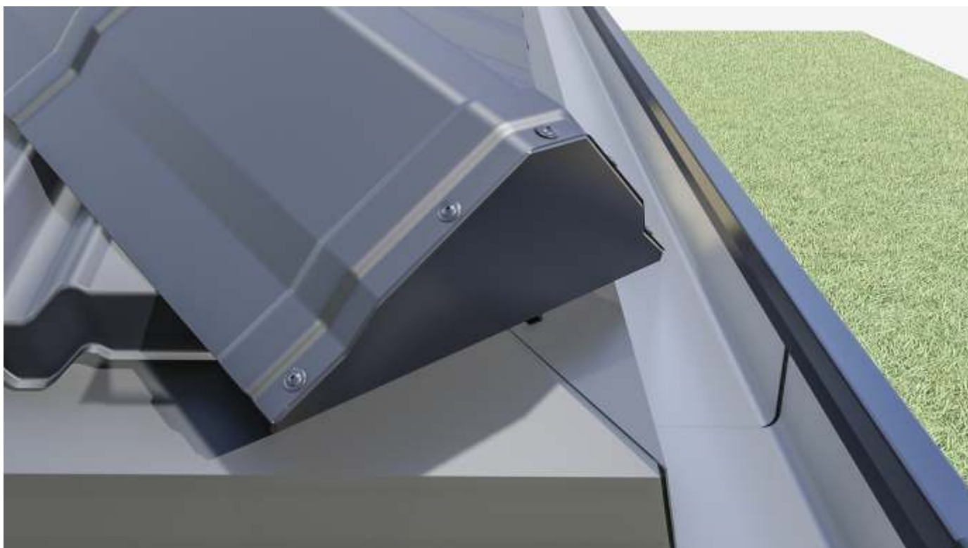
Denko wsunięte w kalenicę i przykręcone za pomocą wkrętów torx.
