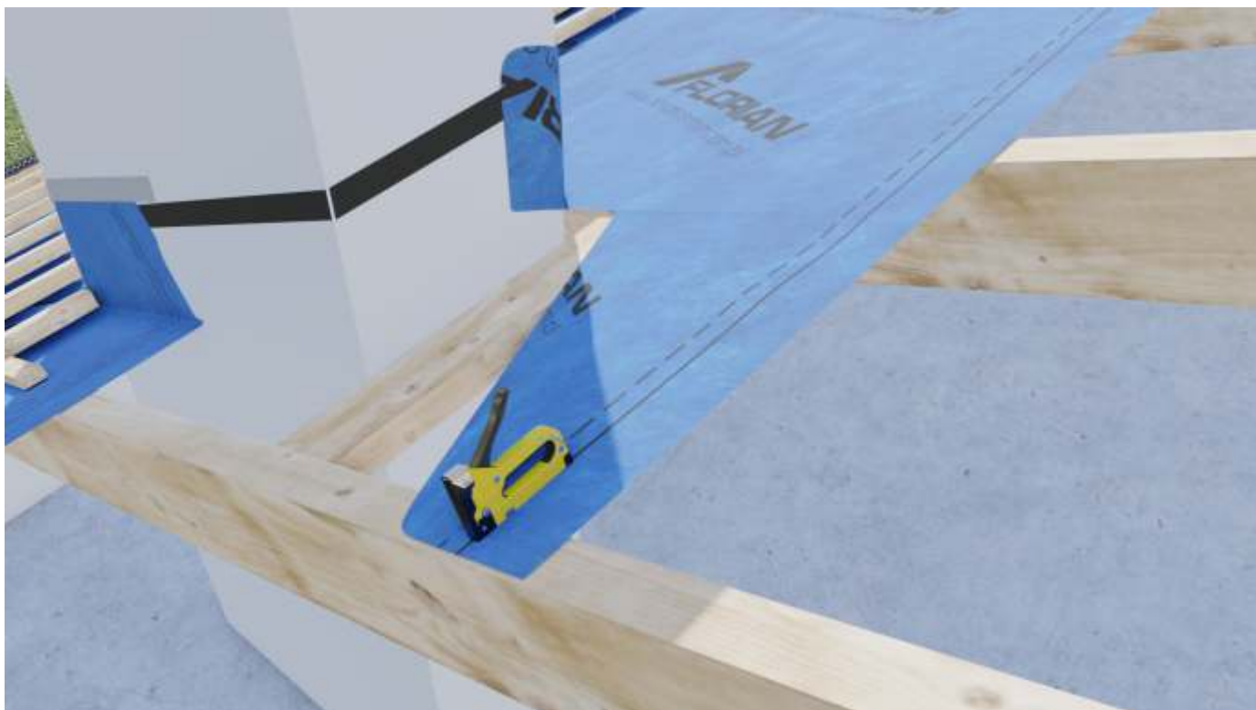
Mocowanie membrany do krokwii za pomocą zszywek.
